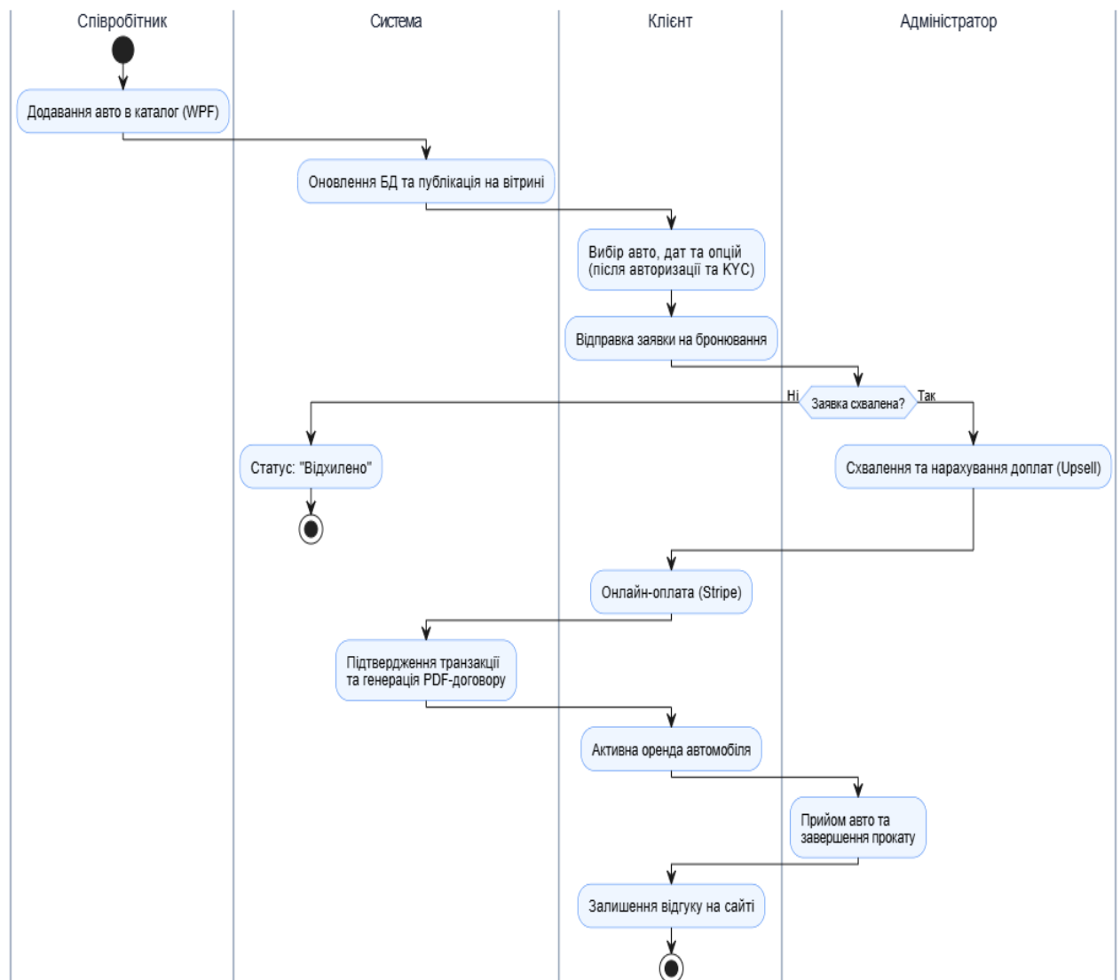
Рисунок 2.9 – Блок-схема узагальненого алгоритму роботи програмного продукту
