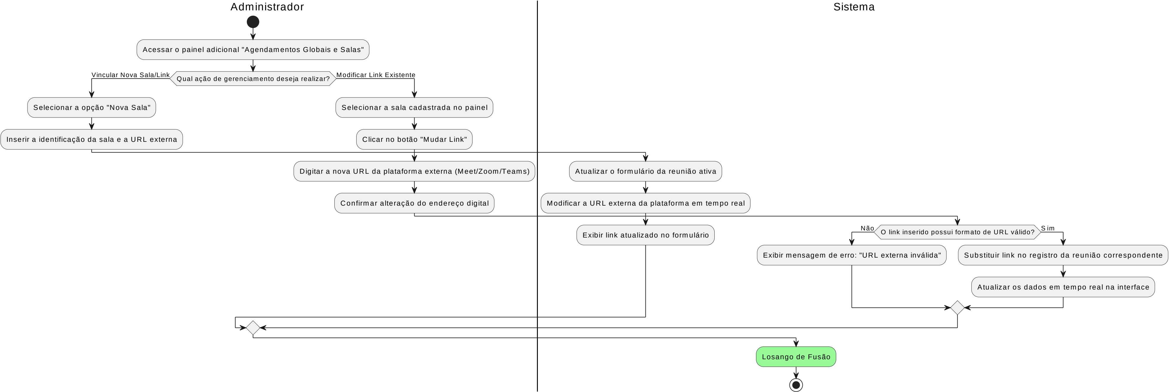
Diagrama de Atividade - Gerenciar Sala (Fiel ao UC12_A3)
