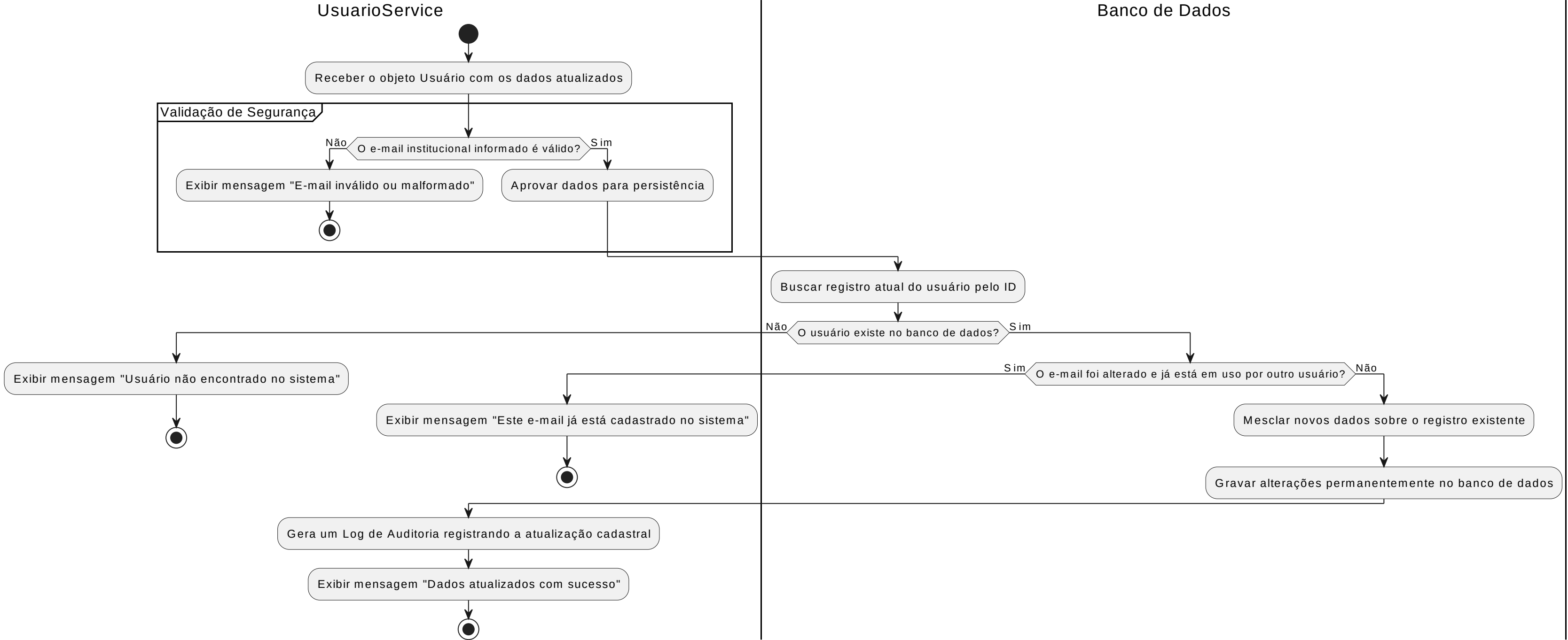
Diagrama de Atividade - Atualizar Registro de Usuário
