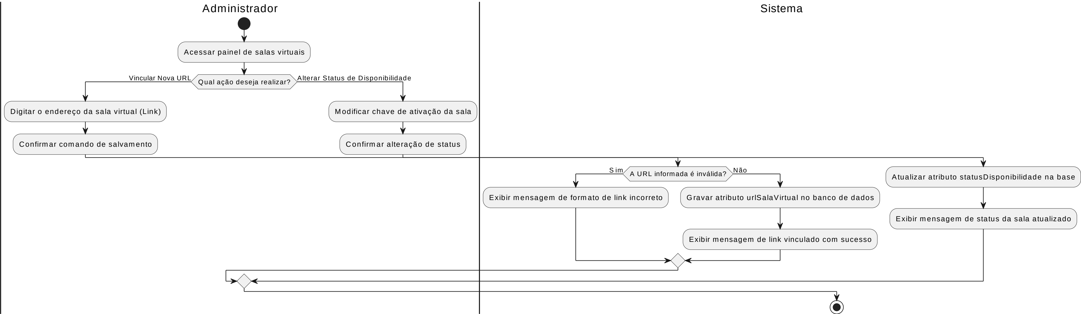
Diagrama de Atividade - Gerenciar Sala (Virtual)
