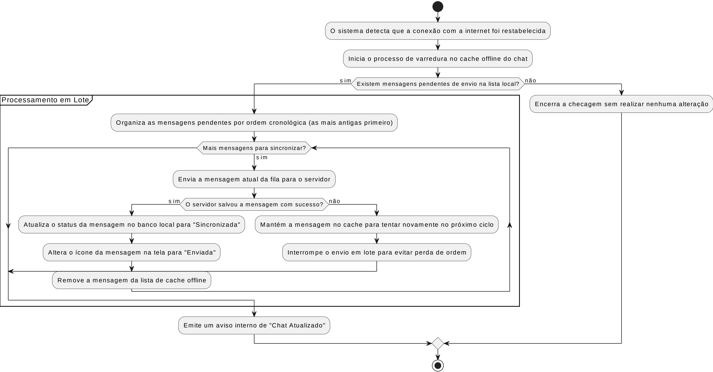
Diagrama de Atividade - Lógica de sincronizarDadosServidor()
