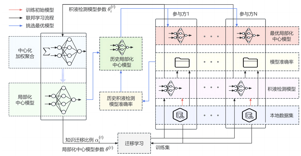
图 4-2 局部化中心模型方案联邦学习训练流程
