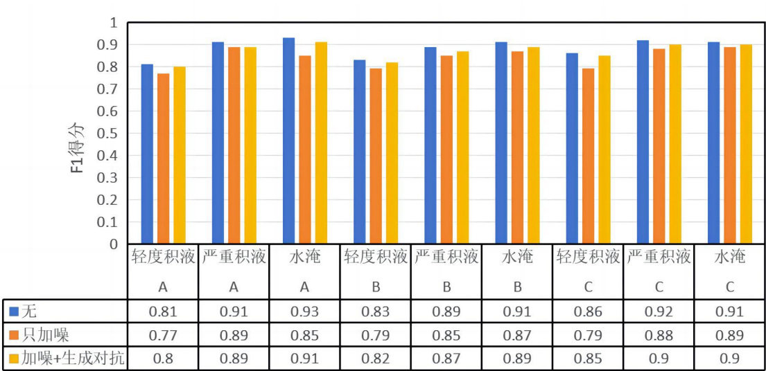
图 5-2 不同加噪方式下三个数据集测试集实验结果
