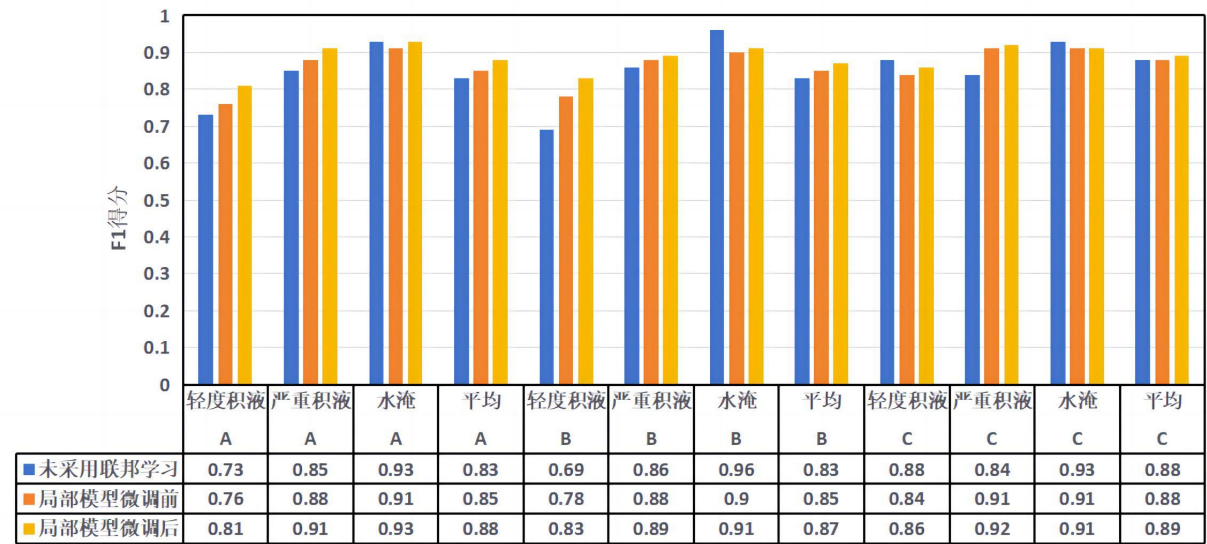
图 4-4 三个数据集测试集上微调前后的 F1 得分（不包括正常数据）
