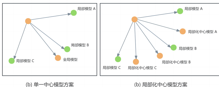
图 4-1 单一中心模型与局部化中心模型（局部模型表示不同区块上的积液检测模型）
