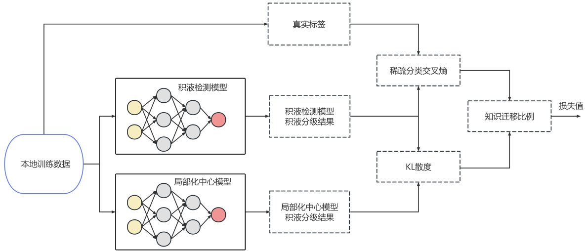
图 4-3 中心模型知识迁移流程图
