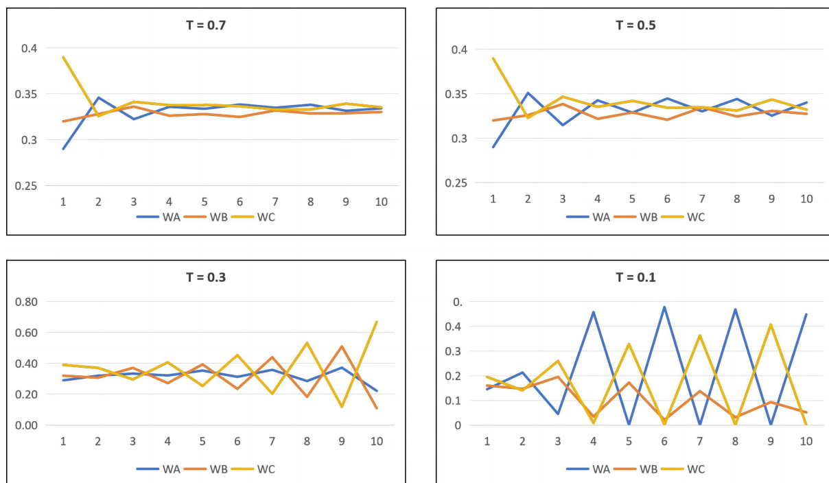
图 4-6 不同温度下三个数据集上局部模型的聚合权重变化
