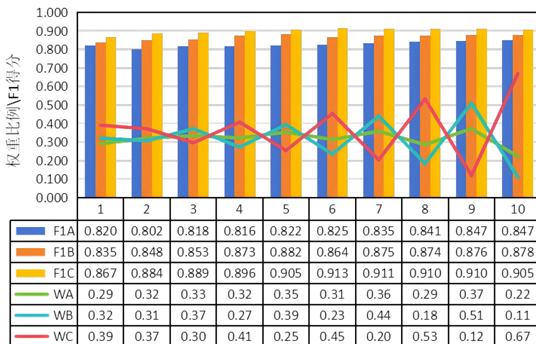
图 4-5 训练过程中三个数据集上局部模型的聚合权重变化及验证集上 F1 得分（不包括正常数据）
