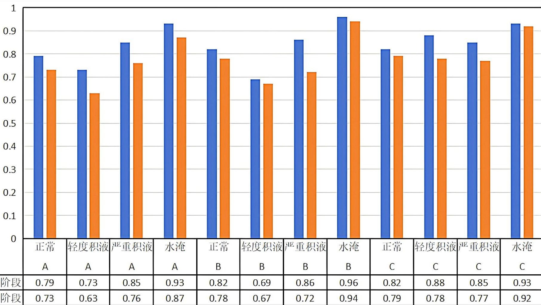
F1得分
