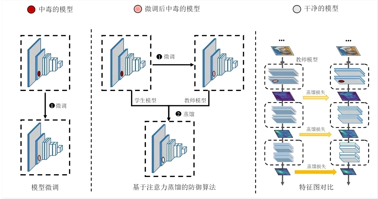
图 5-1 基于注意力蒸馏的防御算法流程 [41]
