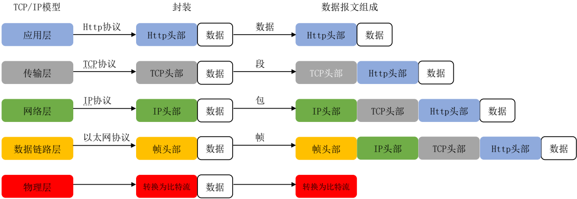
图 2-1 数据封装流程
