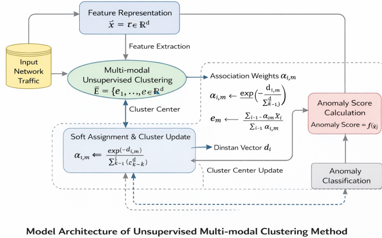
图 4-2 无监督多模式聚类模型架构图
