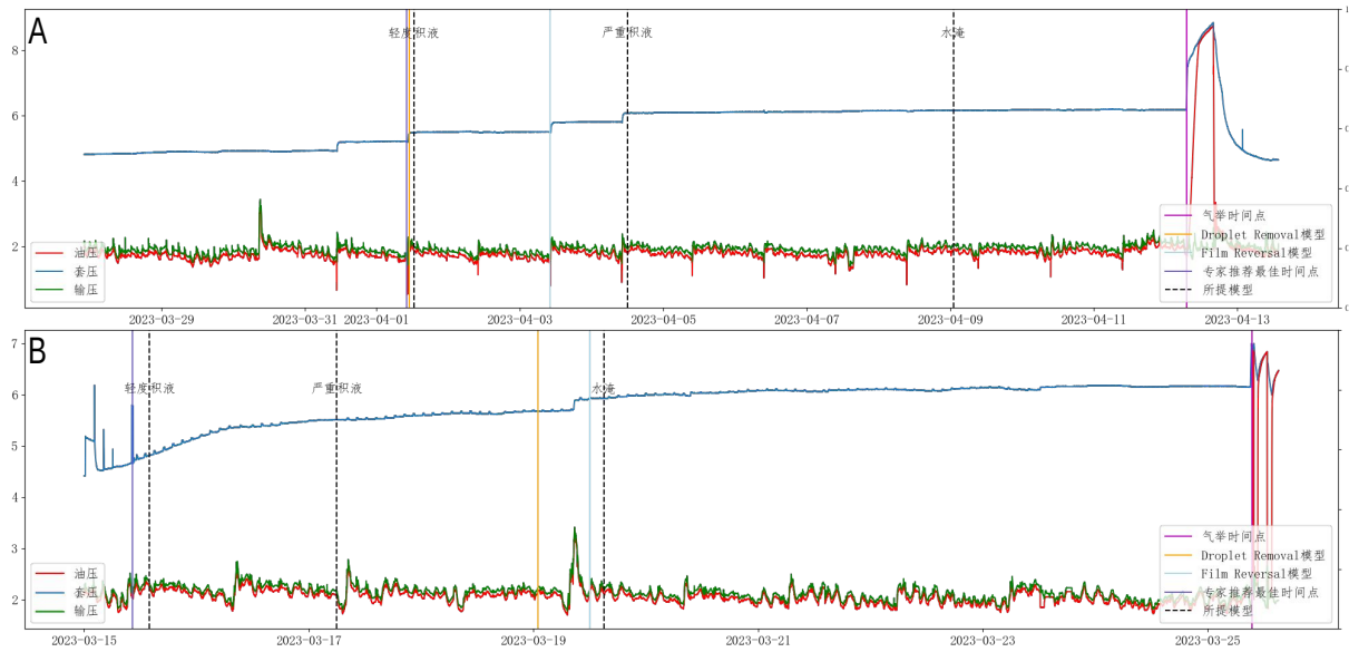
图 3-12 不同模型在自喷井上的积液预警时间点
