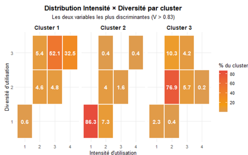
FIGURE 3.15. Distribution intensité et diversité d'utilisation par cluster
