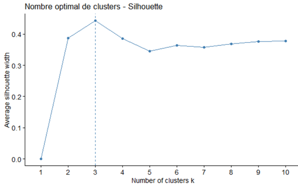
FIGURE 3.13. Coefficient de silhouette selon le nombre de classes
