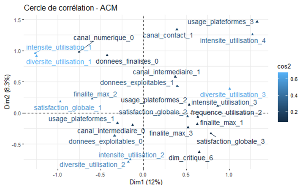
FIGURE 3.11. Cercle de corrélation des variables
