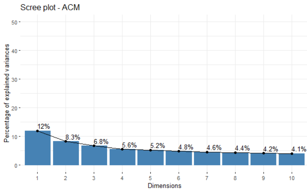
FIGURE 3.10. Diagramme des valeurs propres (scree plot)
