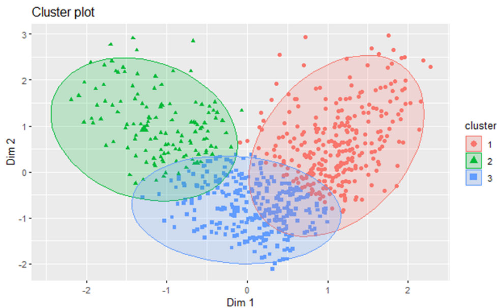
FIGURE 3.14. Visualisation des clusters issus du k-means
