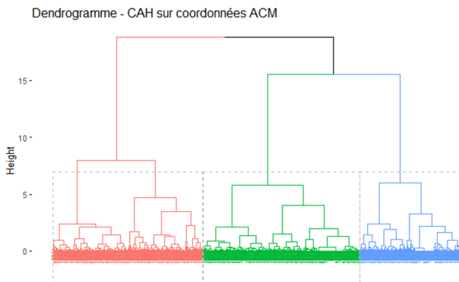
FIGURE 3.12. Dendrogramme de la CAH
