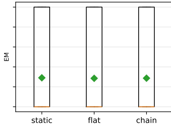
MuSiQue
