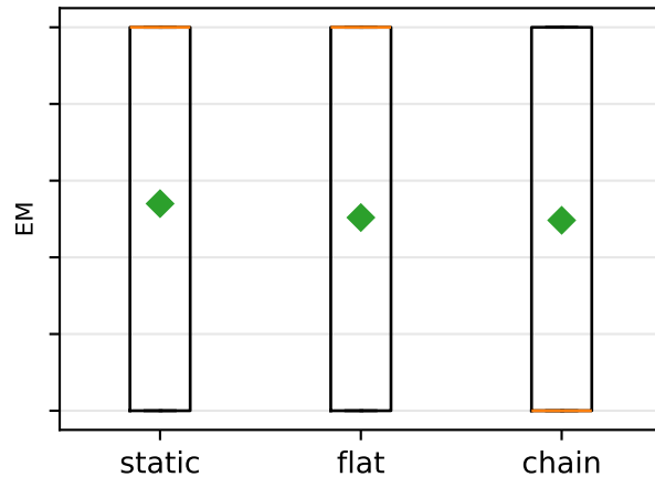
2Wiki
