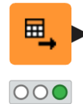
CSV Reader
