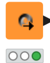
JSON Reader
