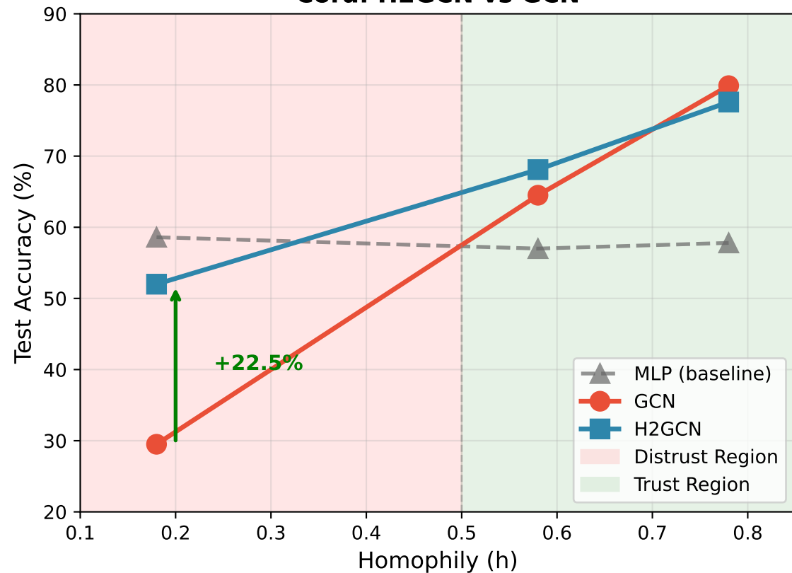
Cora: H2GCN vs GCN
