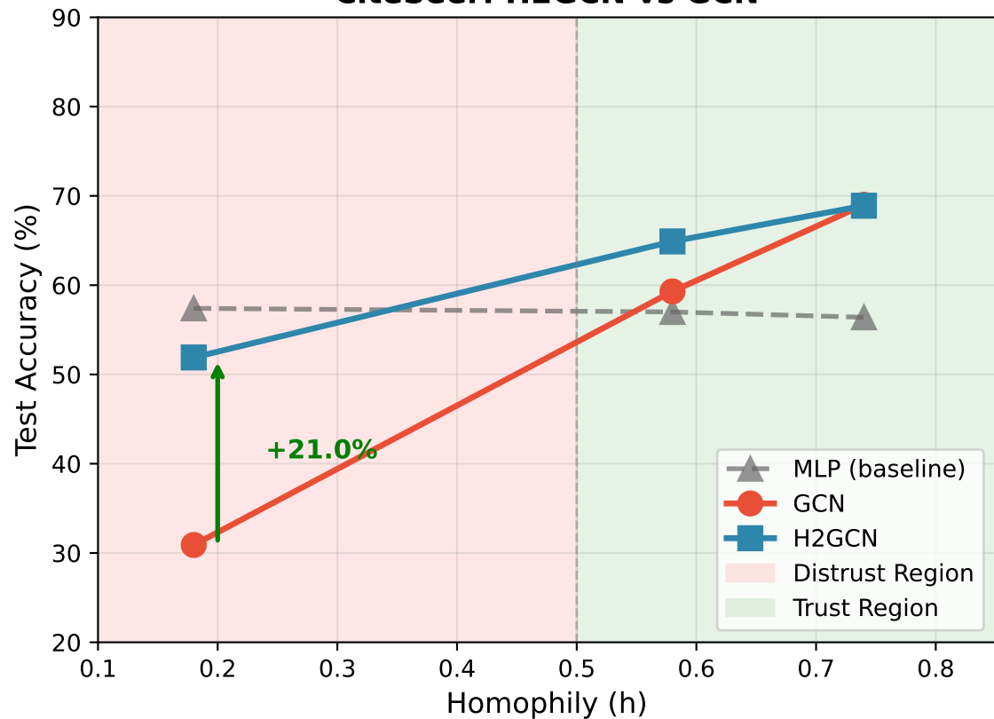
CiteSeer: H2GCN vs GCN
