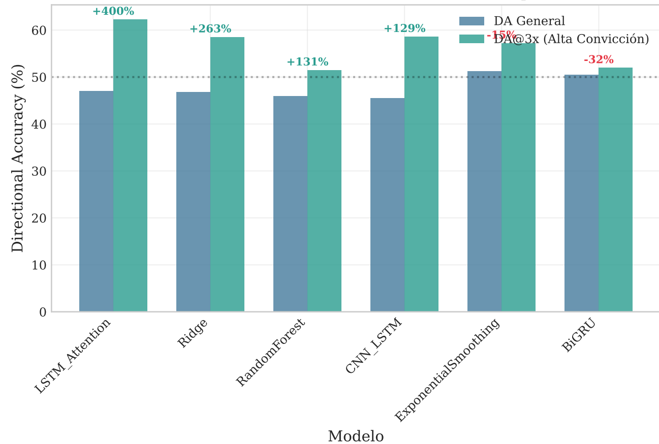
DA General vs DA@3x: Lo Que Realmente Importa
