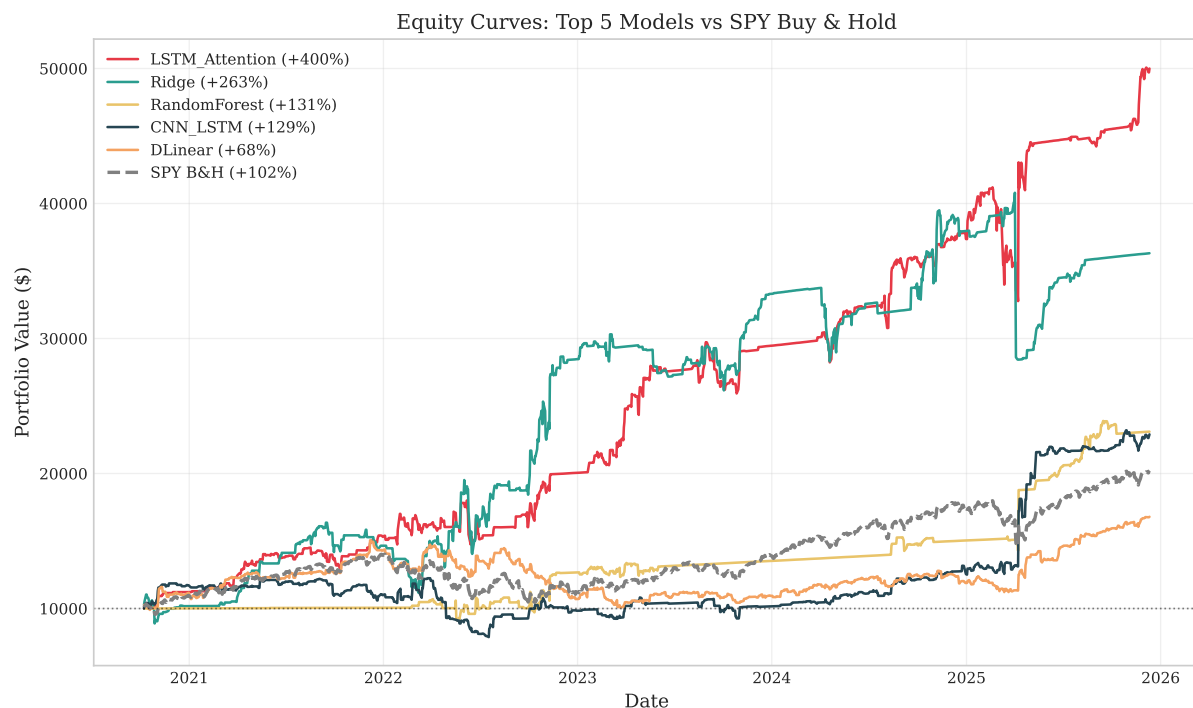
Figura 2: Curvas de equity de los cinco mejores modelos vs SPY Buy & Hold (Oct 2020 – Dic 2025, capital inicial $10,000).
