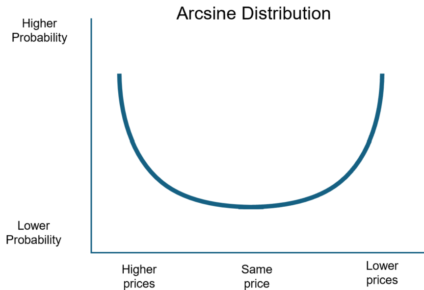
Figura 1: Distribución del arcoseno—la probabilidad de que un camino aleatorio permanezca en territorio de precios altos o bajos es mucho mayor que la de oscilar simétricamente alrededor del precio inicial, generando tendencias persistentes de manera natural. Fuente— CMT Association (2020) .
