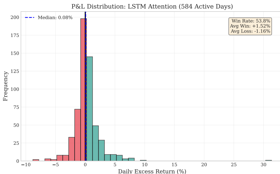
Figura 3: Distribución de retornos diarios en exceso sobre la tasa libre de riesgo del modelo LSTM+Attention. Histograma calculado sobre los días activos (posición \neq 0 ). Verde = días ganadores, Rojo = días perdedores. Línea vertical en 0 %.
