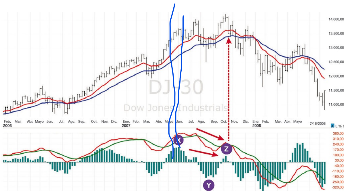
FIGURA 23.4 DJIA semanal, MME de 26 y 13 días, líneas MACD 12-26-9 e histograma MACD (Gráfico de TC2000 en el libro Two Roads Diverged: Trading Divergences ).
