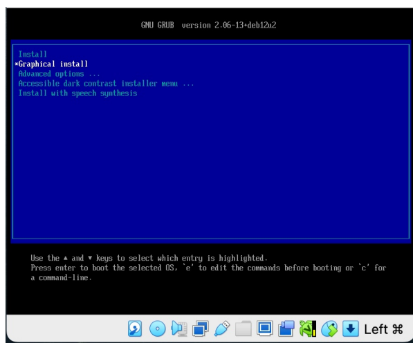
Рис. 3: Окно выбора установщика ОС
