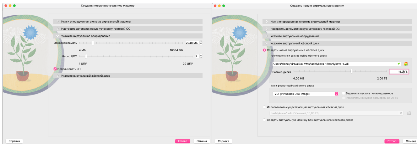
Рис. 2: Выделение оперативной памяти и дискового пространства
