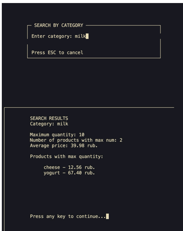
Рис. 21: Поиск по существующей категории
