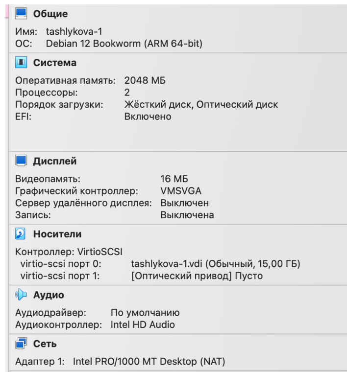
Рис. 8: Детали виртуальной машины
