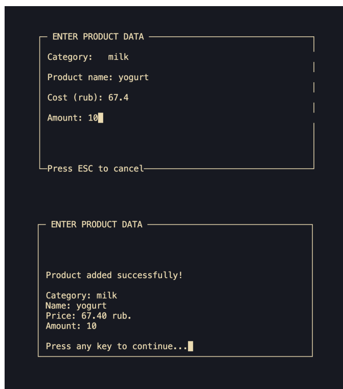
Рис. 16: Добавление нового продукта
