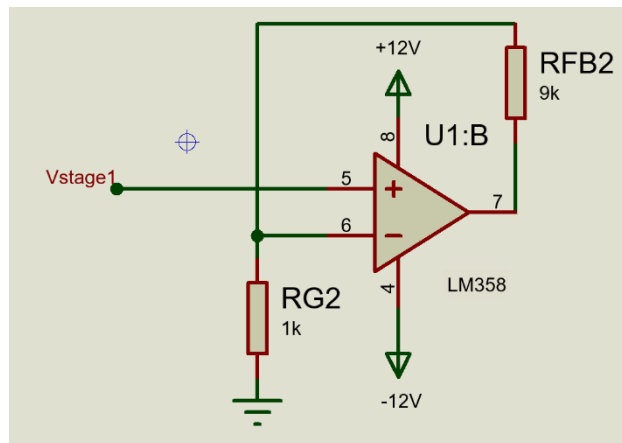
图 3-5：二级放大电路
