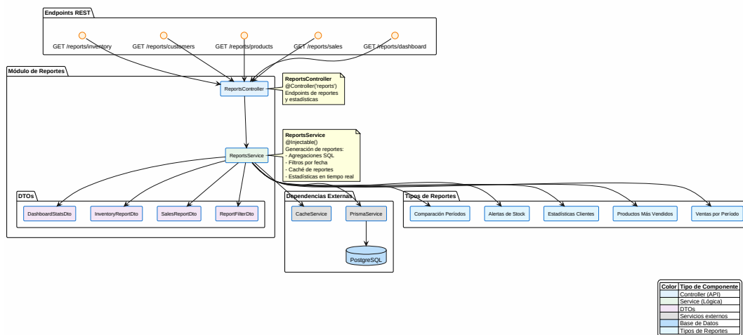
Fig. 12 Diagrama de Componentes - Módulo de Reportes
