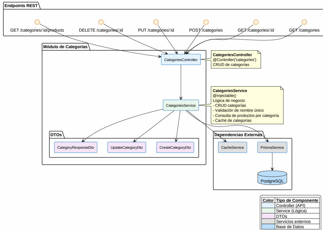
Fig. 15 Diagrama de Componentes - Módulo de Categorías
