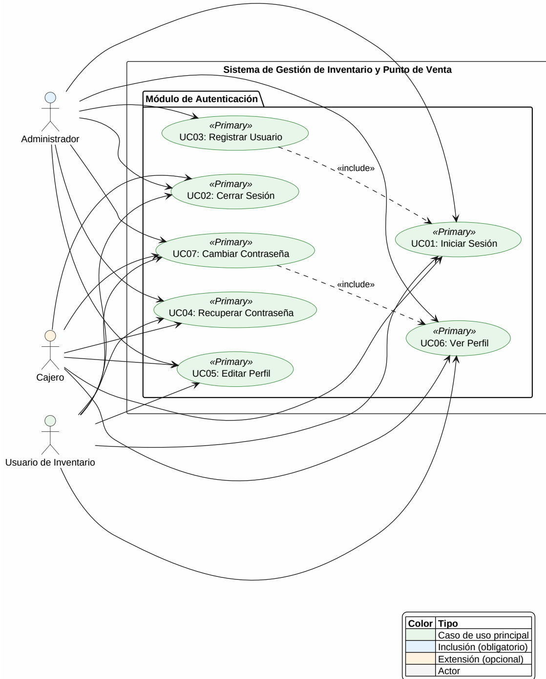
Fig. 1 Diagrama de Casos de Uso - Módulo de Autenticación
