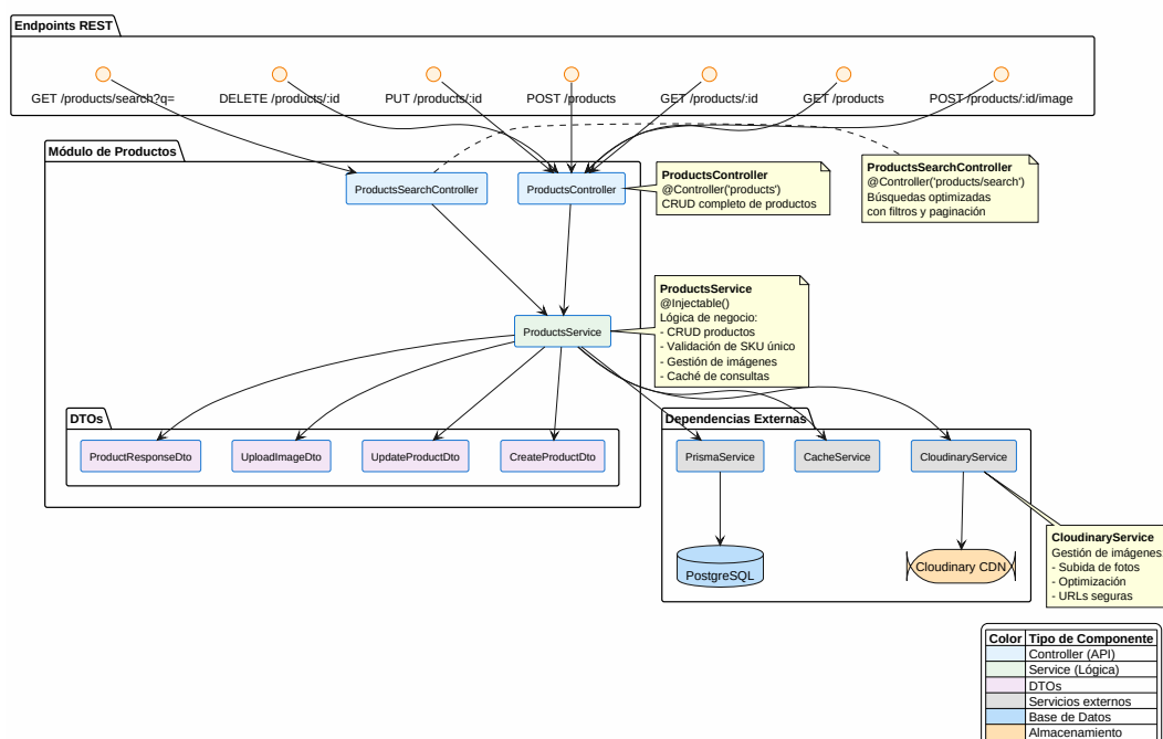
Fig. 9 Diagrama de Componentes - Módulo de Productos
