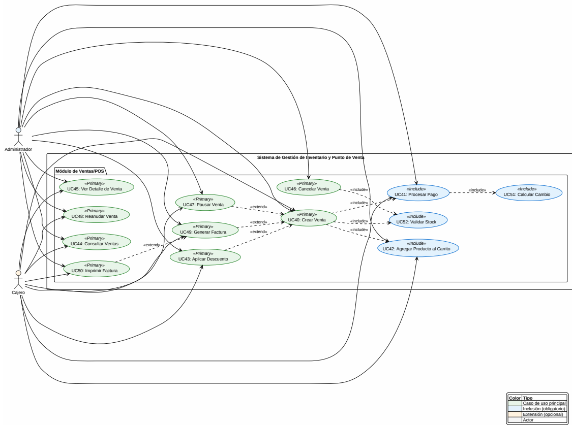
Fig. 3 Diagrama de Casos de Uso - Módulo de Ventas
