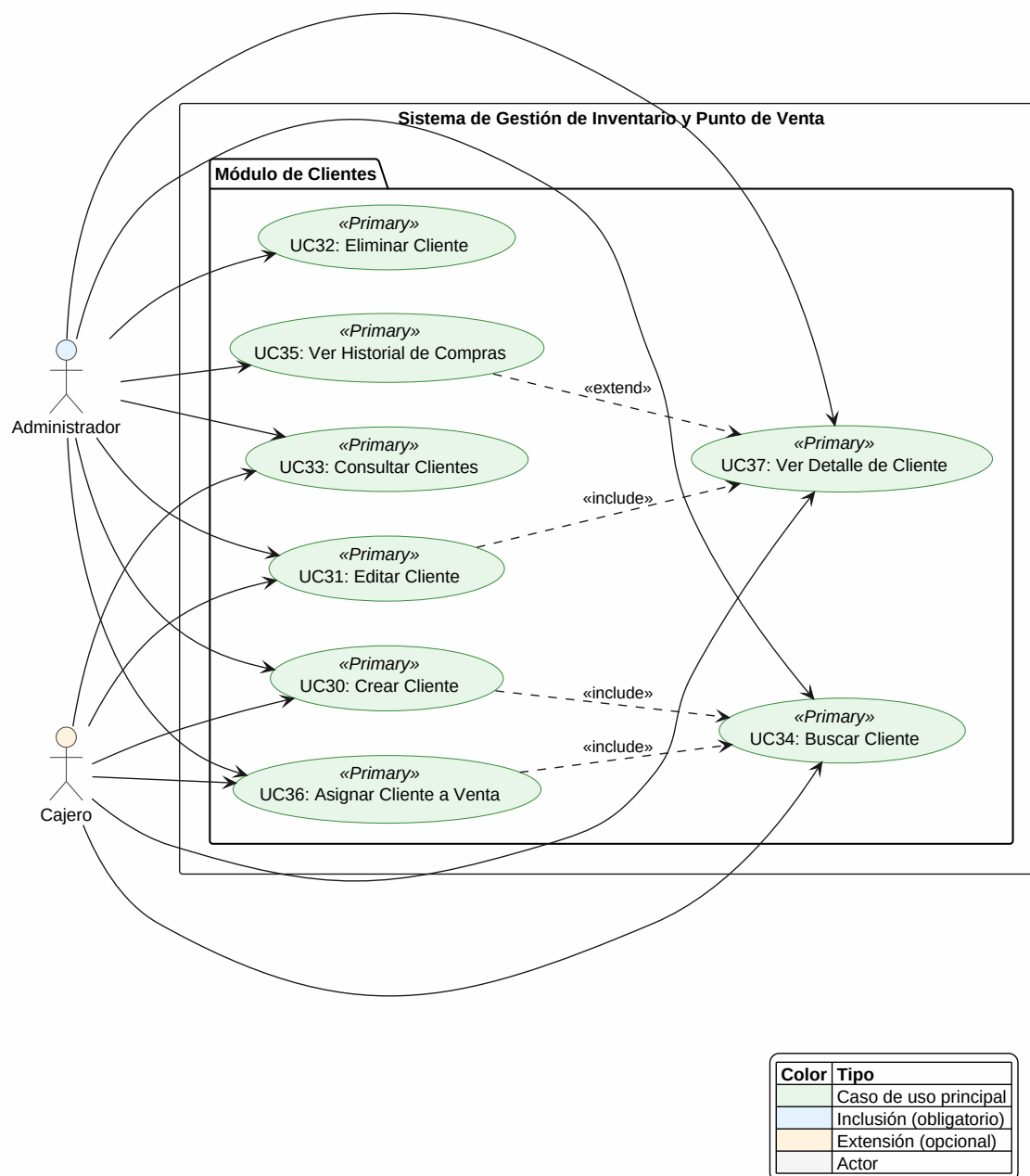
Fig. 4 Diagrama de Casos de Uso - Módulo de Clientes
