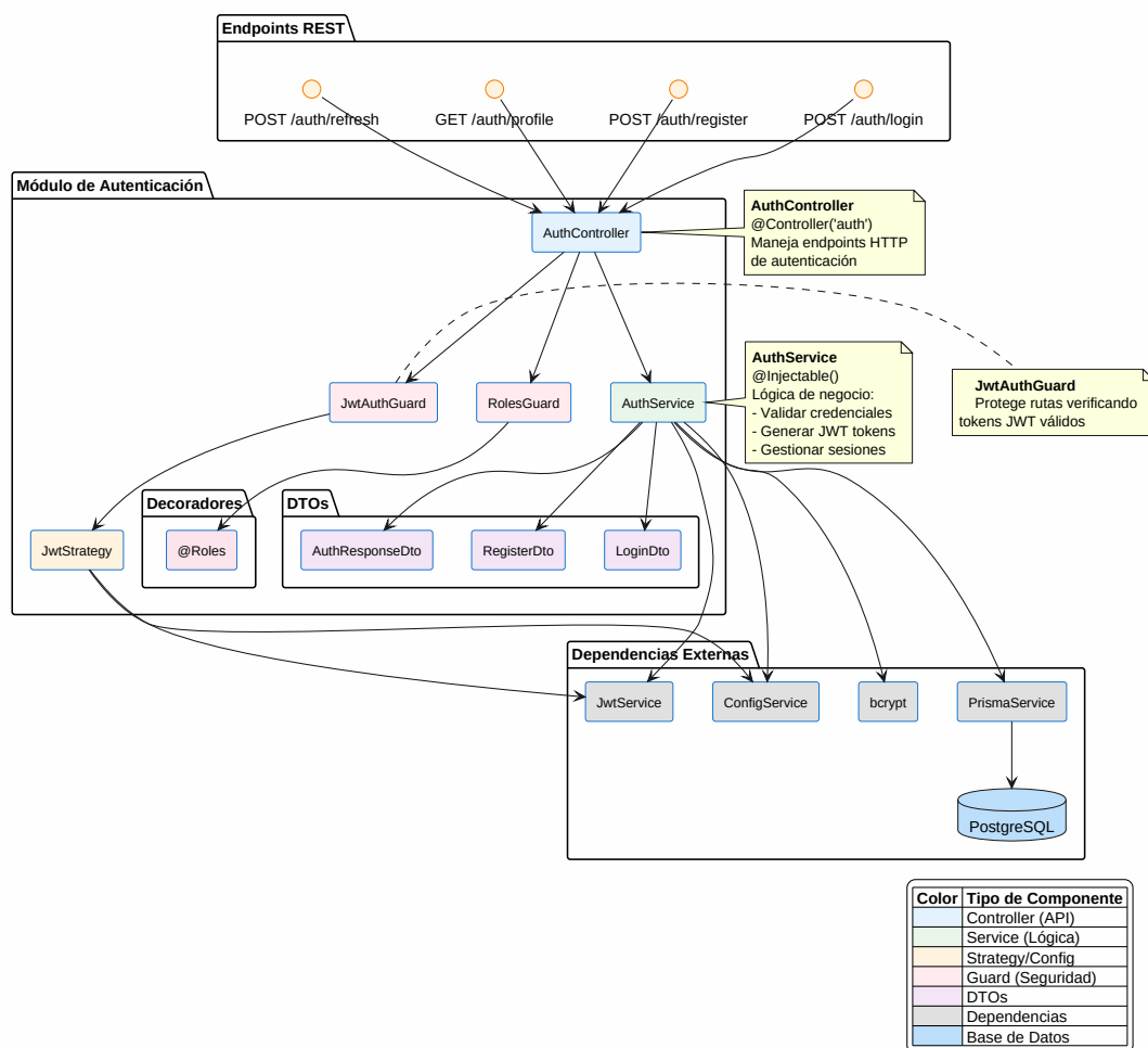
Fig. 8 Diagrama de Componentes - Módulo de Autenticación
