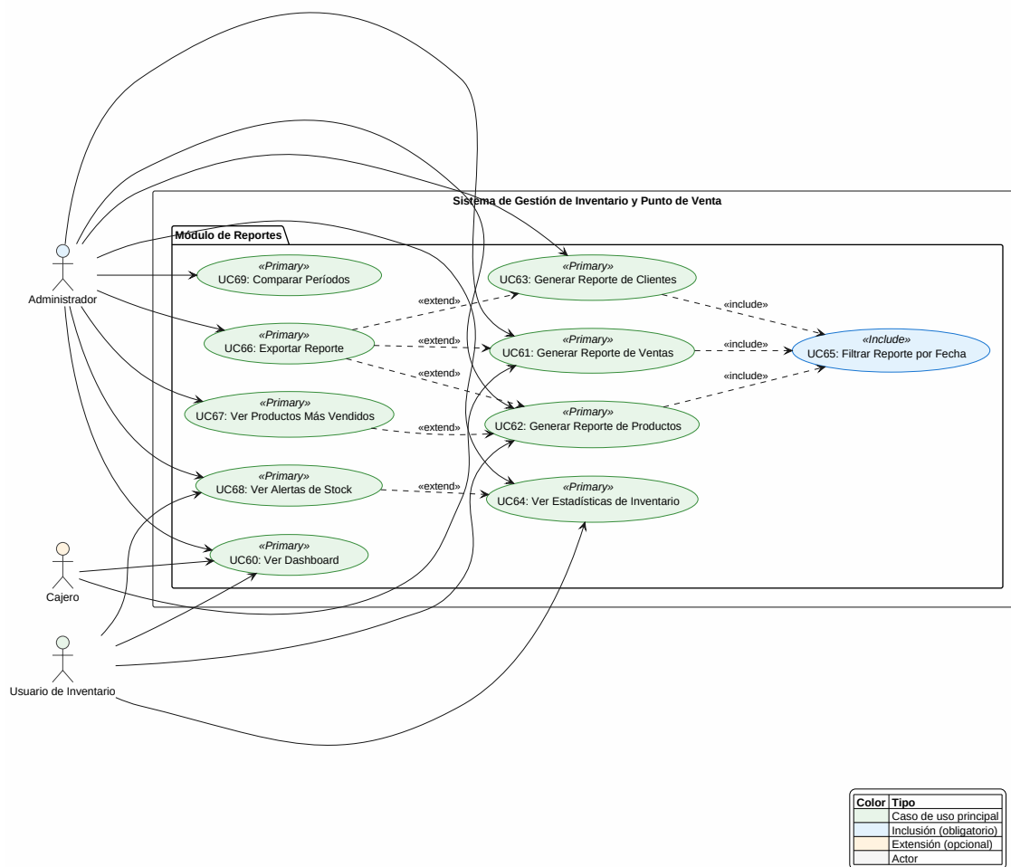
Fig. 5 Diagrama de Casos de Uso - Módulo de Reportes
