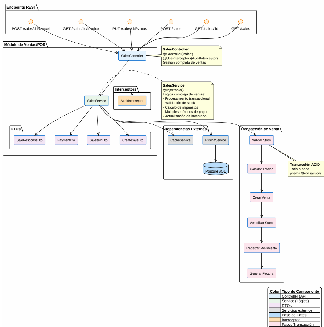
Fig. 10 Diagrama de Componentes - Módulo de Ventas
