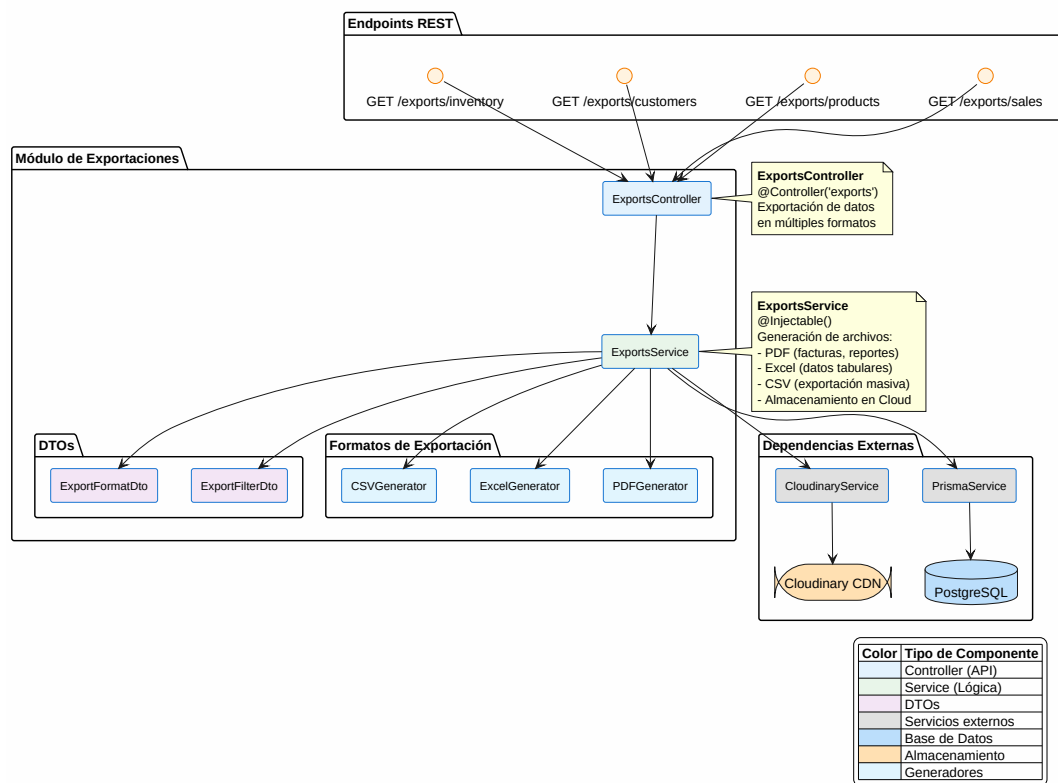
Fig. 13 Diagrama de Componentes - Módulo de Exportaciones
