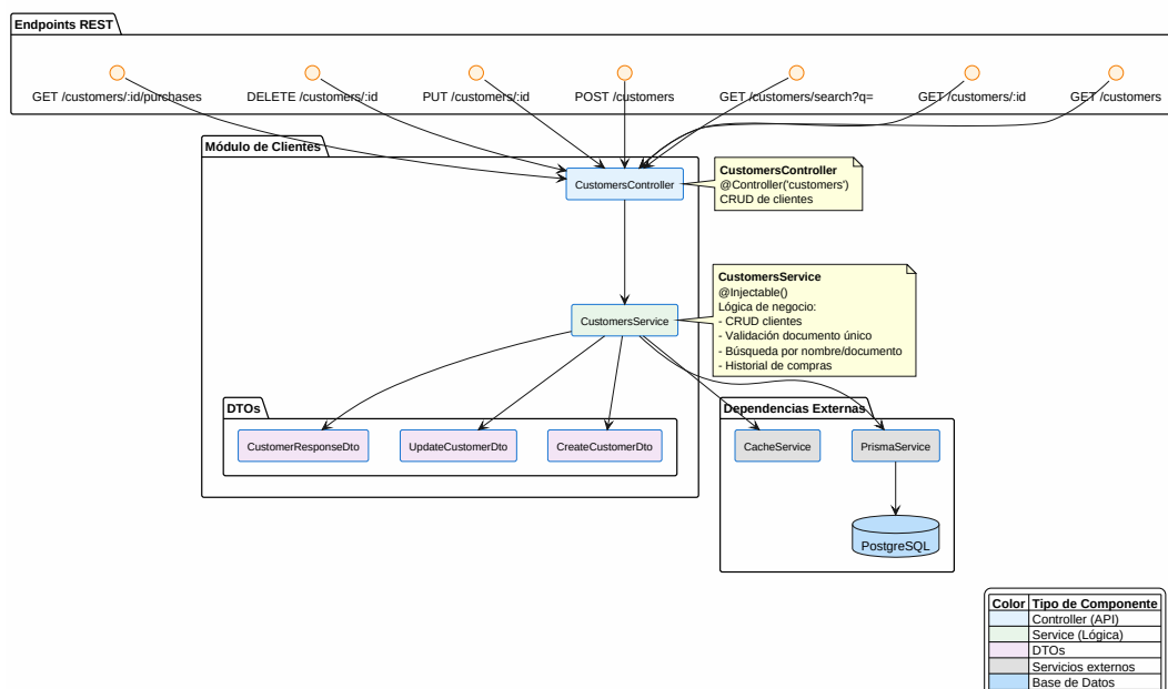
Fig. 11 Diagrama de Componentes - Módulo de Clientes
