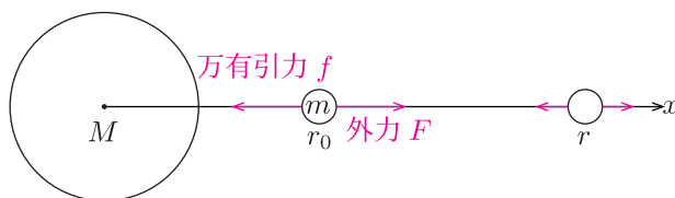
Fig.3 万有引力と外力が働く物体
