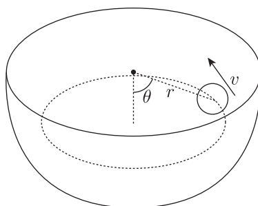
Fig.5 お椀の中で等速円運動する小球
