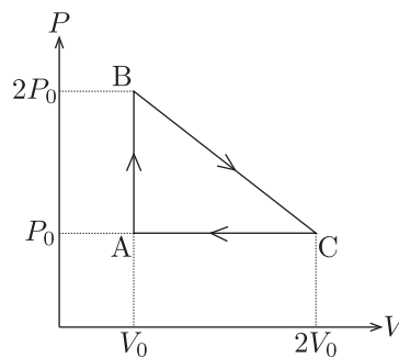
Fig.20 P-V グラフ
