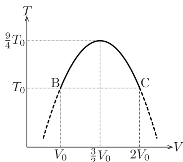
Fig.22 T - V グラフ
