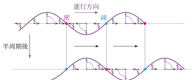
Fig.3 右向きに進行する疎密波。右方向の振動の変位を鉛直上向きとした。
