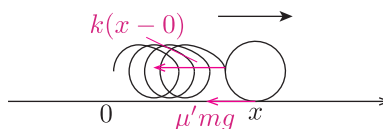
Fig.20 力の図示
