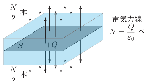
Fig.11 帯電した平板から出る電気力線とガウス面
