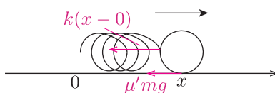
Fig.20 力の図示
