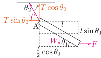
Fig.4 力の図示
