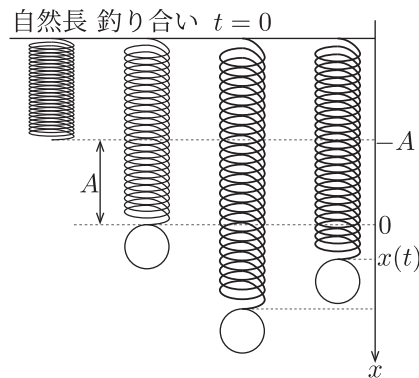
Fig.5 鉛直ばねの単振動
