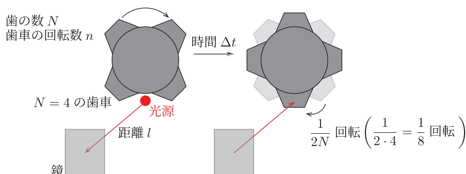
Fig.29 回転歯車による光速測定実験
