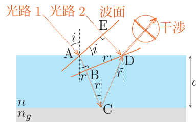
Fig.62 薄膜へ光波の斜方入射による反射光の干渉
