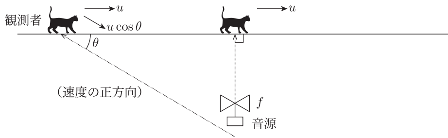
Fig.13 音源と観測者が角度をなす場合
