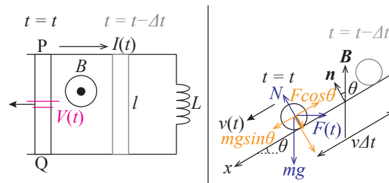
Fig.42 回路図と導体棒に働く力
