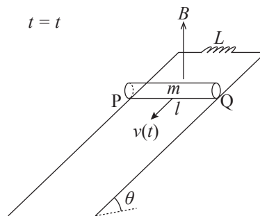
Fig.41 任意の時刻 t = t における斜面上を運動する導体棒 (ソレノイド接続)
