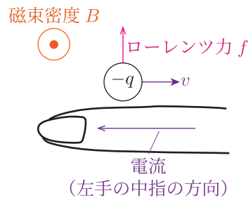
Fig.10 負の荷電粒子が受けるローレンツ力
