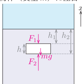
Fig.25 流体中で静止する物体に働く力の図示
