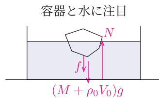
Fig.28 力の図示
