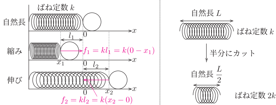
Fig.1 フックの法則
