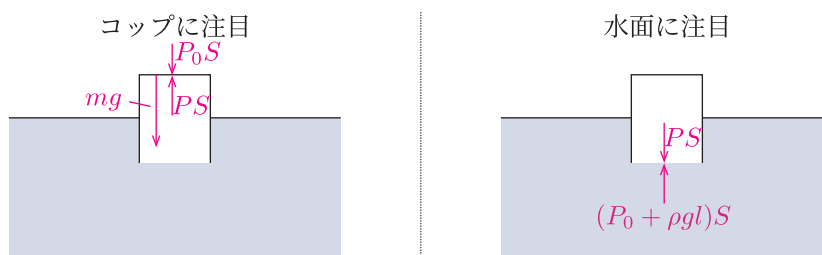
Fig.30 力の図示
