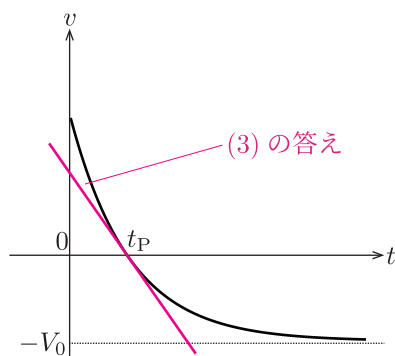
Fig.36 v-t グラフ
