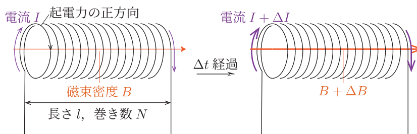
Fig.3.35 ソレノイドに流れる電流の時間変化
