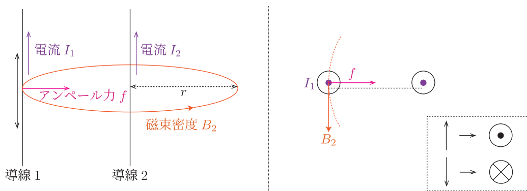
Fig.8 2つの直線電流
