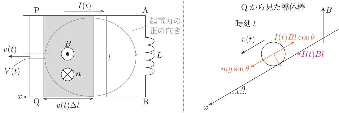
Fig.43 回路図と導体棒に働く力
