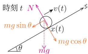
Fig.17 力の図示
