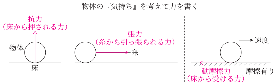
Fig.10 接触力の具体例
