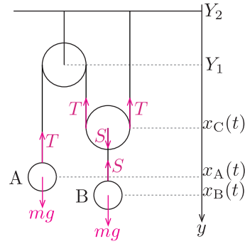
Fig.26 力の図示
