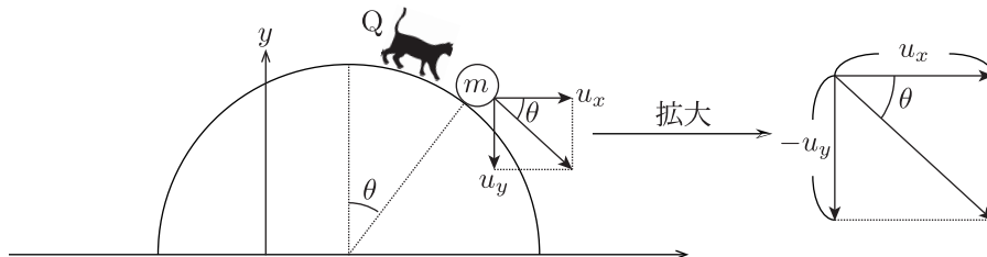
Fig.28 Q からみた小球の速度
