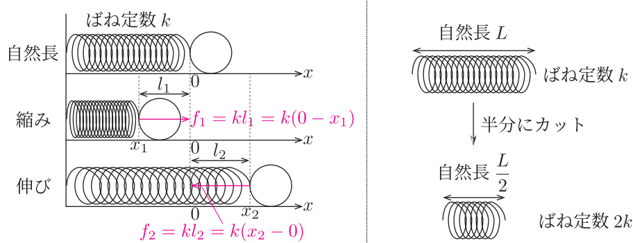
Fig.27 フックの法則
