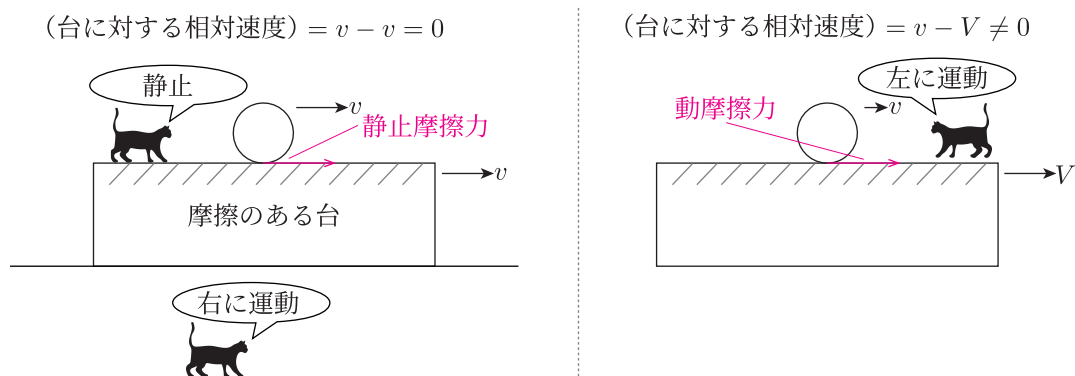
Fig.33 静止摩擦力と動摩擦力
