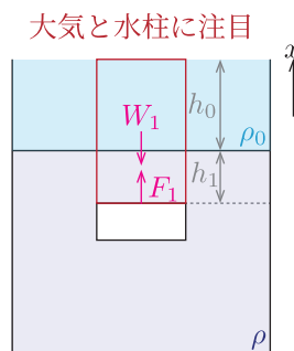
Fig.48 大気と水の柱に働く力の図示
