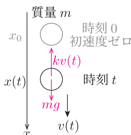
Fig.45 空気抵抗を考慮した落下運動
