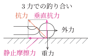
Fig.34 粗い面から受ける抗力
