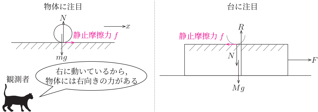
Fig.38 小物体と台に働く力
