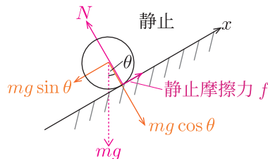
Fig.41 一瞬静止したときの力の図示
