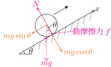
Fig.40 粗い斜面上を運動する物体の力の図示
