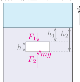
Fig.50 流体中で静止する物体に働く力の図示
