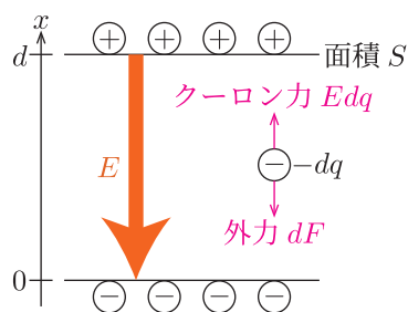
Fig.29 外力により電荷を蓄えるコンデンサー
