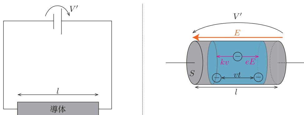
Fig.31 電池に繋がれた導体と導体内の自由電子
