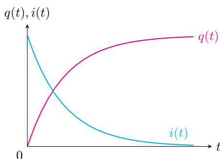
Fig.34 q(t) と i(t) の時間推移
