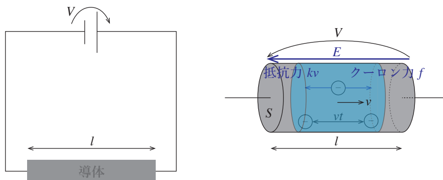
Fig.31 電源に繋がれた導体と導体内の自由電子の様子
