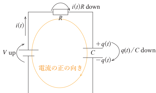
Fig.32 抵抗とコンデンサーの直流回路
