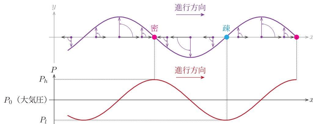
Fig.2 空気の疎密波と圧力波 P - x グラフ
