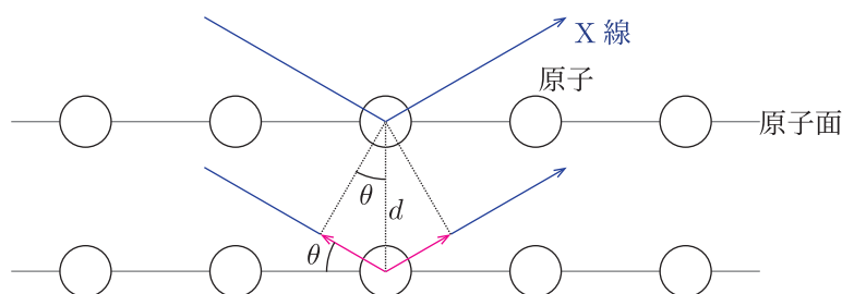
Fig.27 ブラッグ反射の概略図
