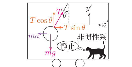
Fig.16 非慣性系による議論
