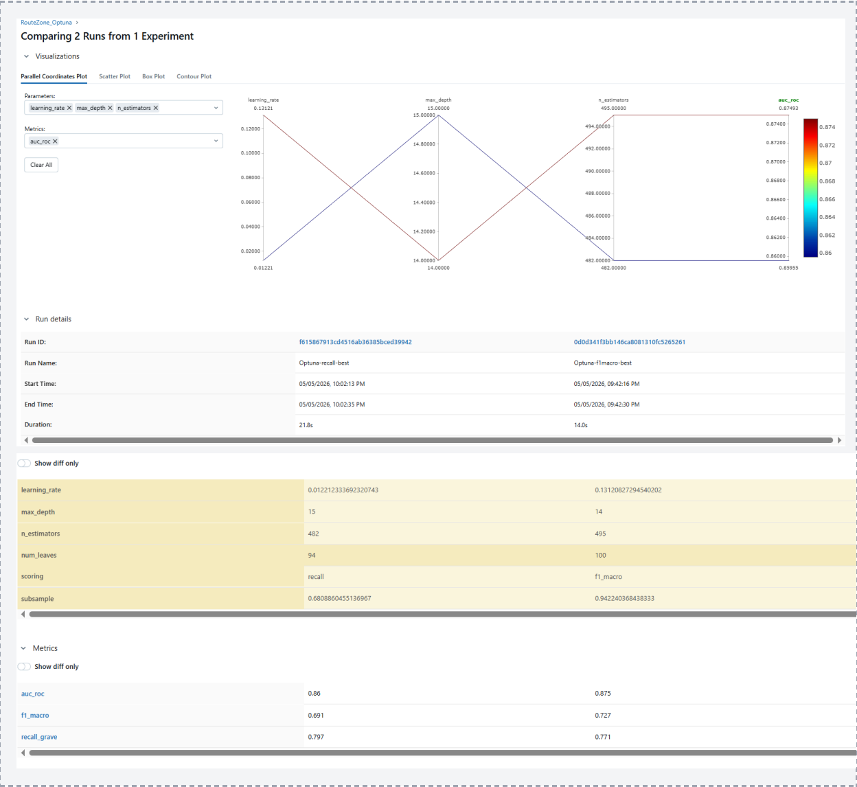
Figure 4 — MLflow UI : comparaison recall et F1 Optuna
