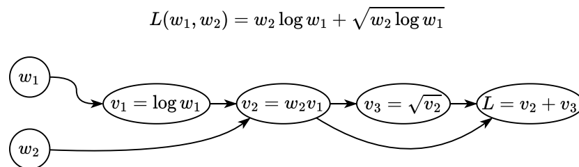
Рисунок 21: Вычислительный граф
