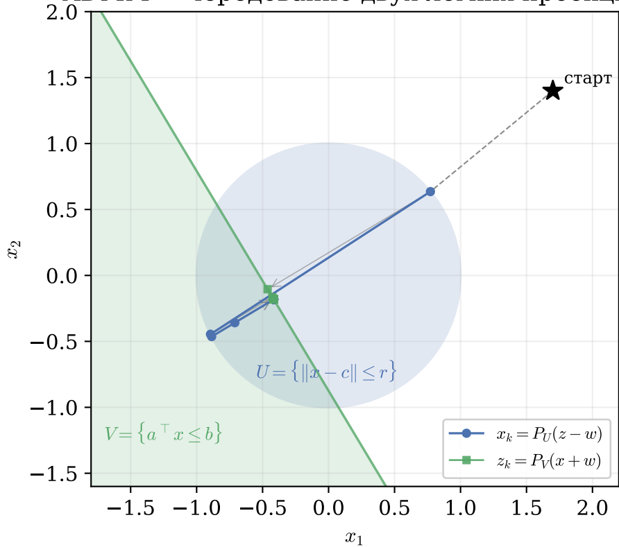
ADMM = чередование двух лёгких проекций
