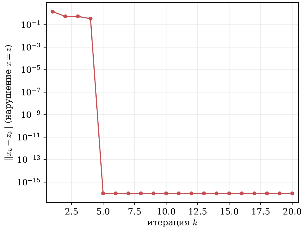
Сходимость к самому пересечению
