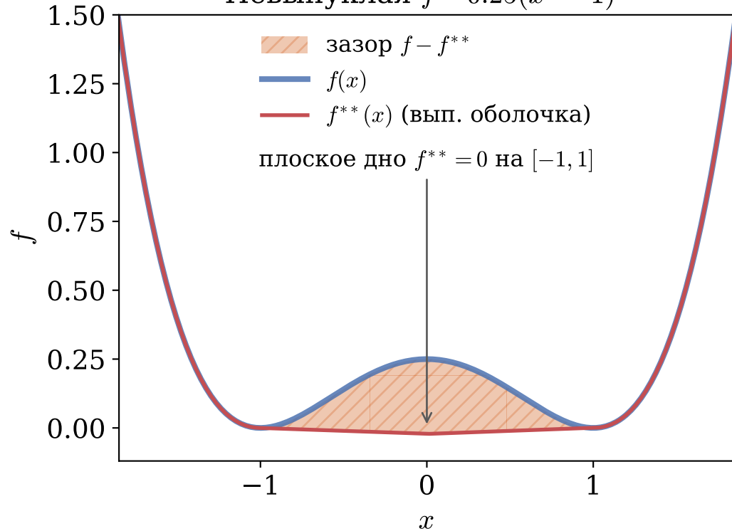
Невыпуклая f = 0.25(x^2 - 1)^2
