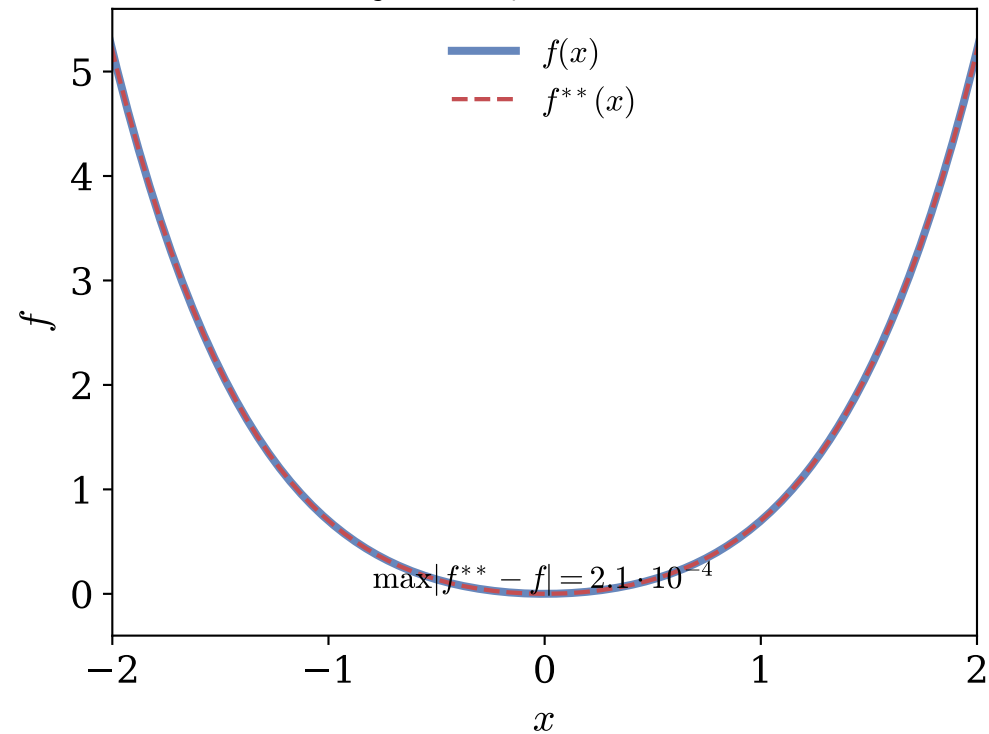
Выпуклая f = 0.5x^2 + 0.2x^4
