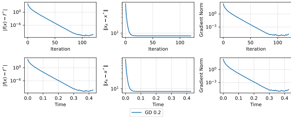
Figure 19: Выпуклая задача не имеет сходимости по аргументу
