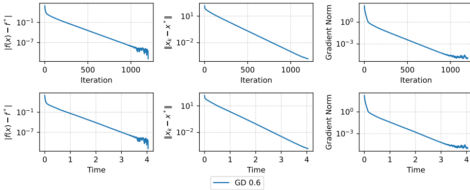
Figure 21: Другой способ обеспечить сходимость в предыдущей задаче - поменять местами значения размерности задачи
