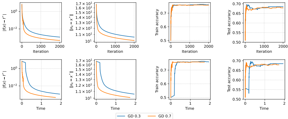
Figure 22: Лишь небольшая точность может быть достигнута с сублинейной сходимостью
