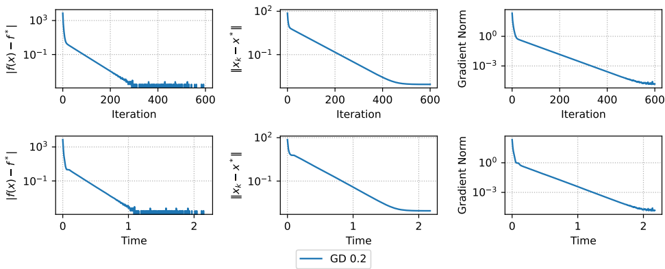
Figure 20: Но если добавить даже небольшую регуляризацию, вы гарантируете сходимость по аргументу
