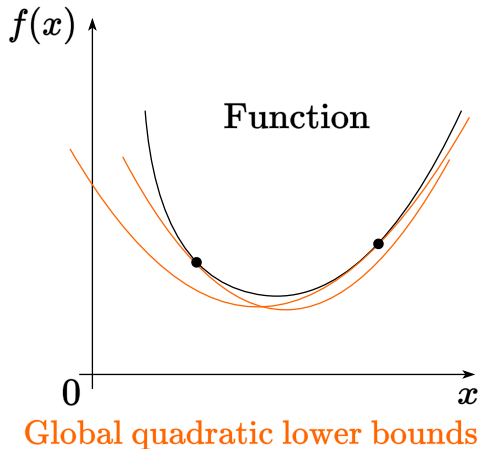
Figure 14: Сильно выпуклая функция не меньше некоторой параболы в любой точке
