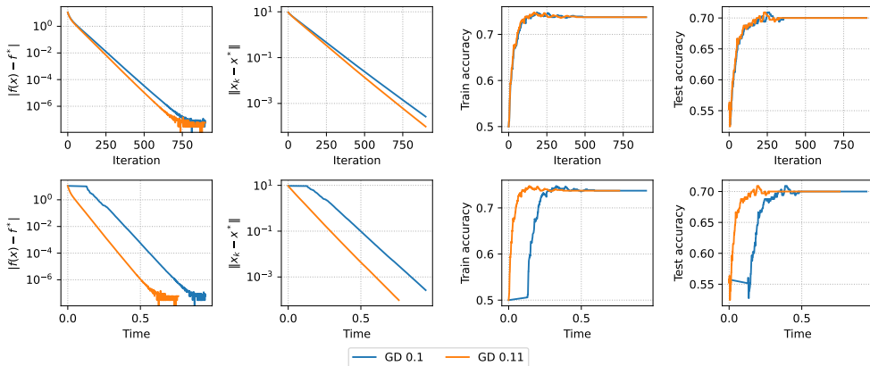
Figure 23: Сильная выпуклость обеспечивает линейную сходимость
