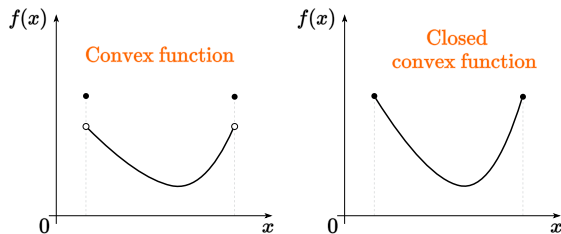
Figure 15: Выпуклые функции могут иметь разрывы на границе своей области определения.
