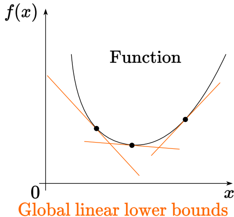
Figure 13: Выпуклая функция больше или равна линейной аппроксимации Тейлора в любой точке
