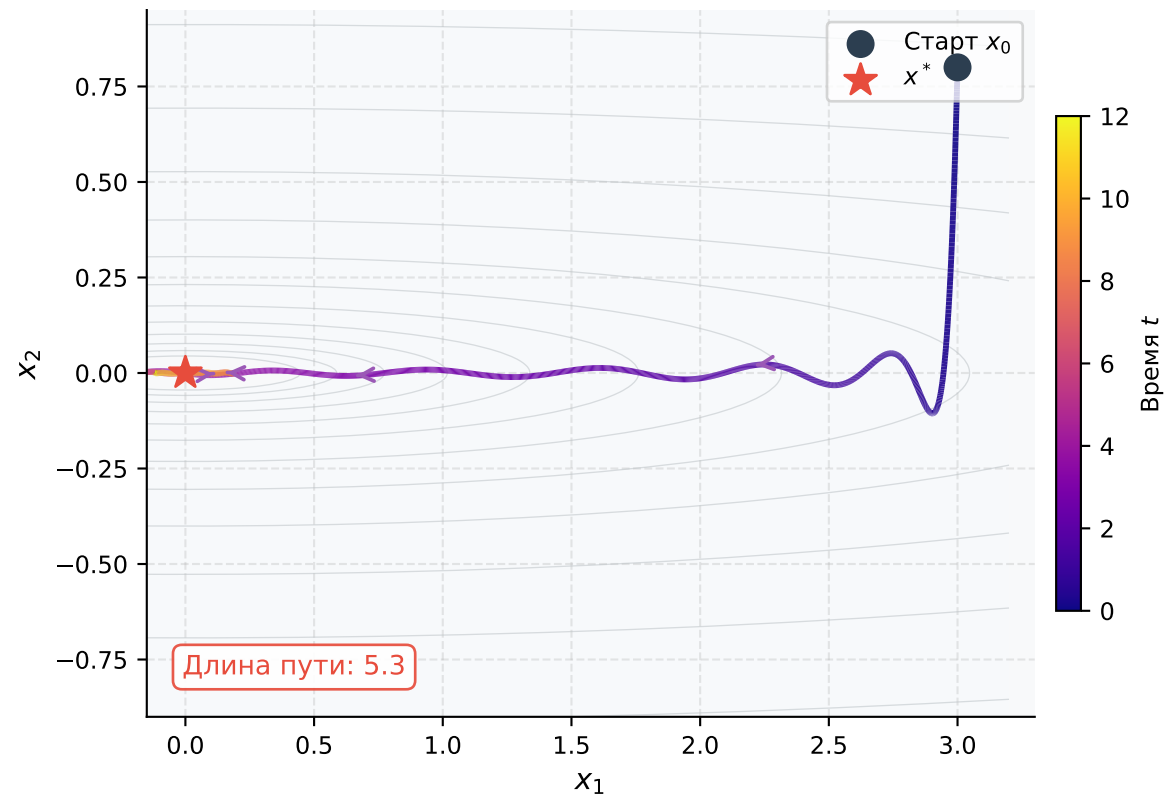
AGF (Нестеров) — зигзаг, \kappa=100
