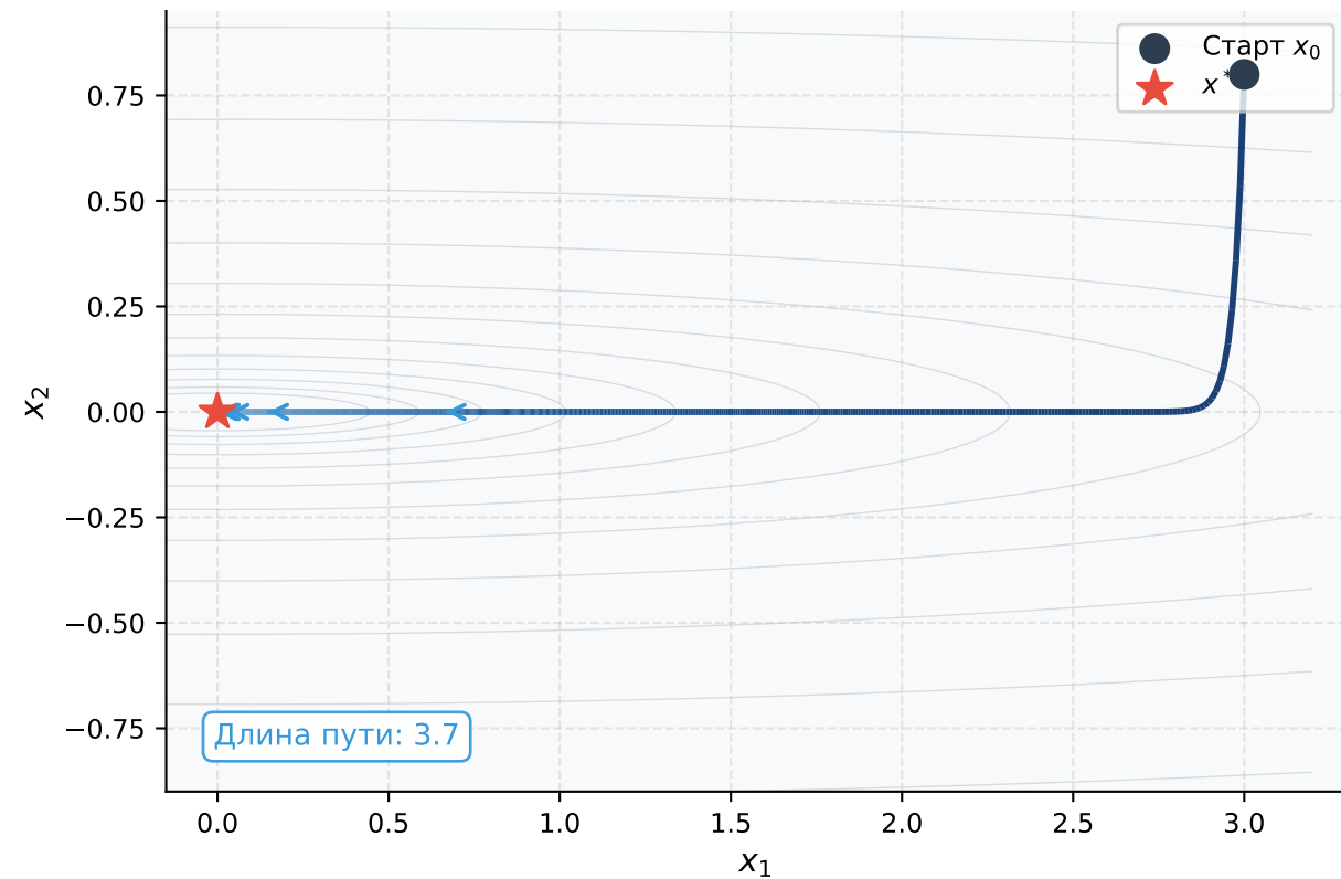
GF — монотонный спуск
