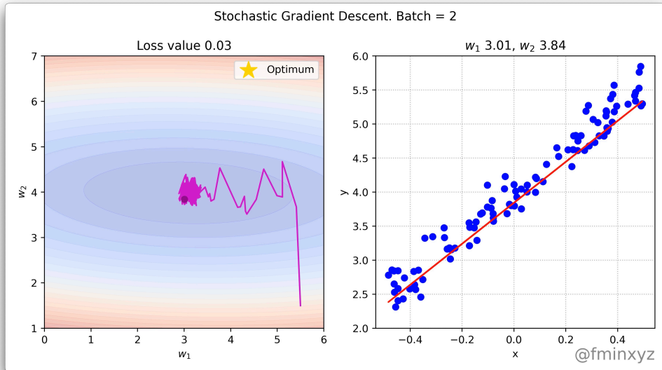
Figure 1: Расходимость SGD при постоянном шаге
