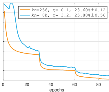
Figure 7: Постоянный warmup
