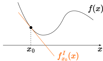
Figure 1: Аппроксимация Тейлора первого порядка в окрестности точки x_0
