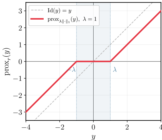
Figure 2: Оператор мягкого порога: «мёртвая зона» [-\lambda, \lambda]
