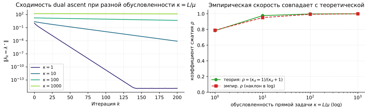
Рис. 2: Слева — сходимость dual ascent для квадратичных задач с разной обусловленностью \kappa = L/\mu . Справа — эмпирический коэффициент сжатия \rho (наклон лог-графика) совпадает с теоретическим (\kappa_d - 1)/(\kappa_d + 1) , где \kappa_d — обусловленность двойственной задачи.
