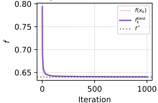
Polyak: немонотонность
