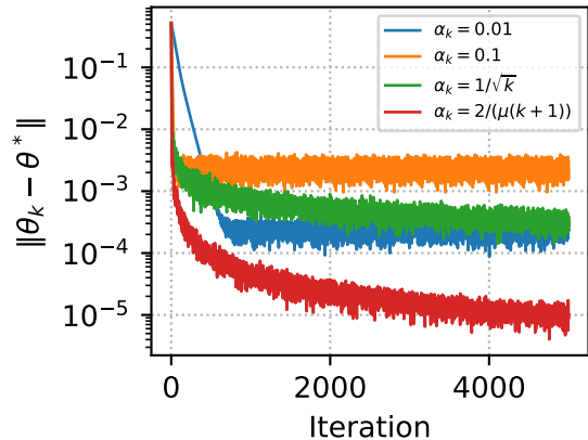
Сходимость по аргументу
