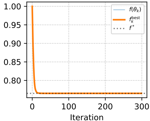
\alpha_k = 0.1 (постоянный шаг)
