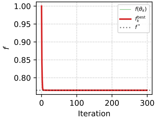
\alpha_k = 1/\sqrt{k} (убывающий шаг)
