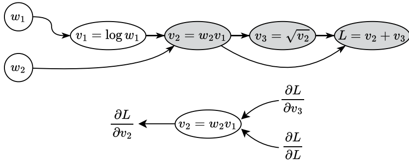
Рис. 23: Иллюстрация обратного режима автоматического дифференцирования
